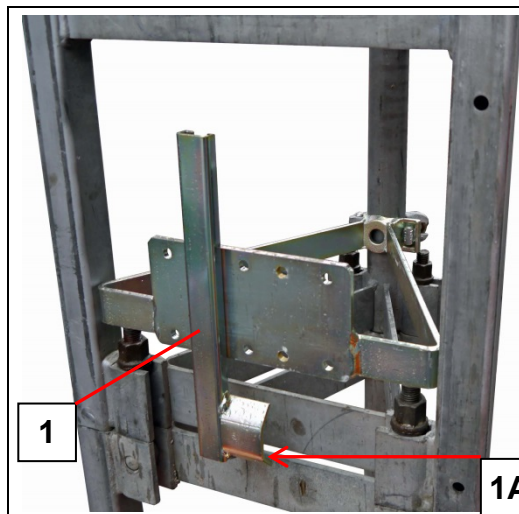
Endschalteranfahrbügel Etage (kurz) für 500 Z/ZP 3
