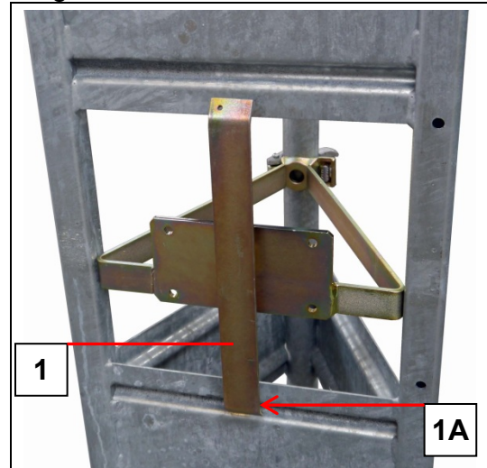
Endschalteranfahrbügel Etage für 500 Z/ZP
