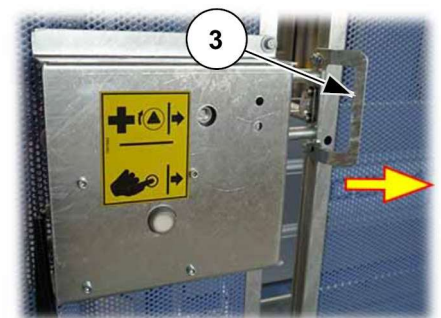
Abb. 42: Schiebetür schließen
