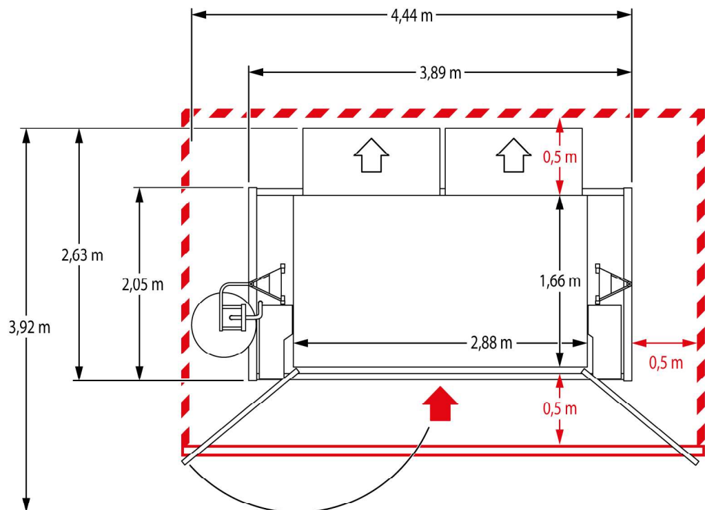
Abb. 19: Platzbedarf Bühne E
