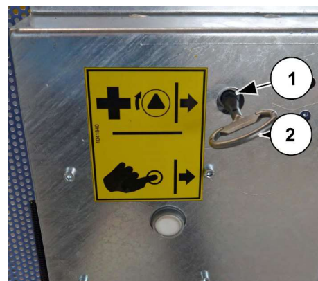
Abb. 44: Schiebetür Notentriegelung von außen
