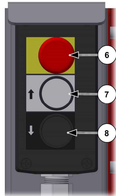
Abb. 62: Steuerung Entladerampe
