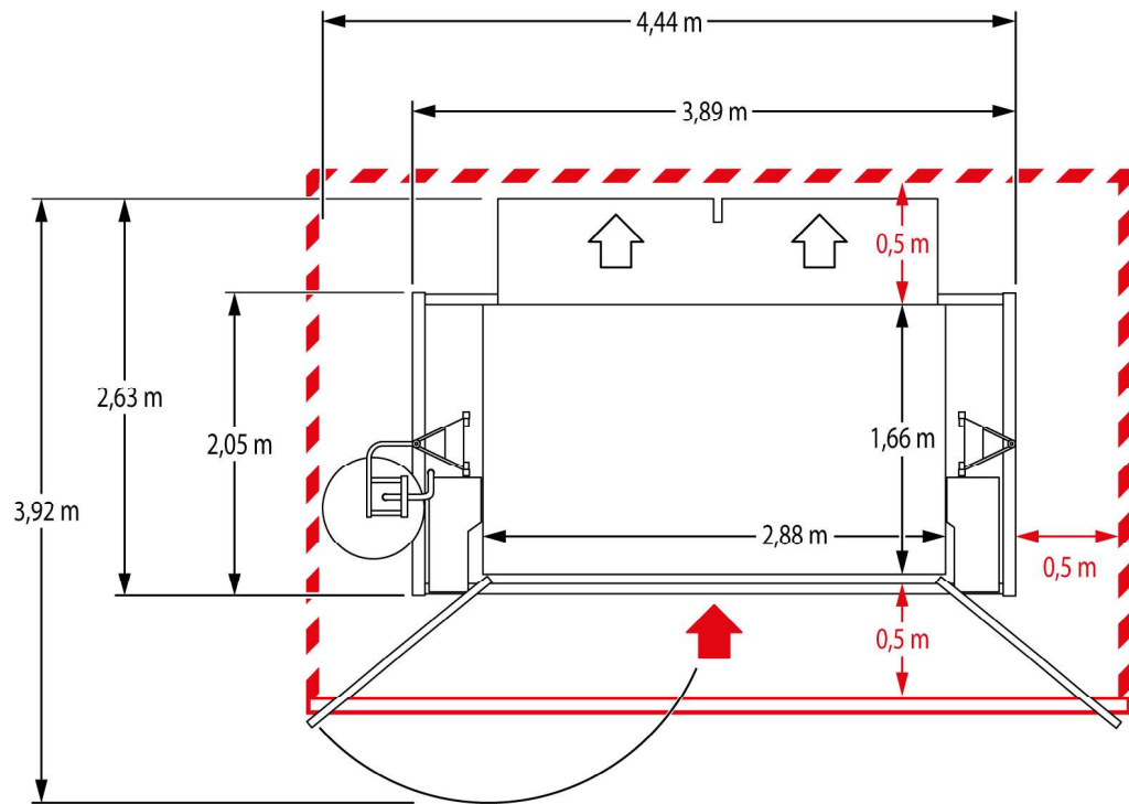
Abb. 21: Platzbedarf Bühne ED
