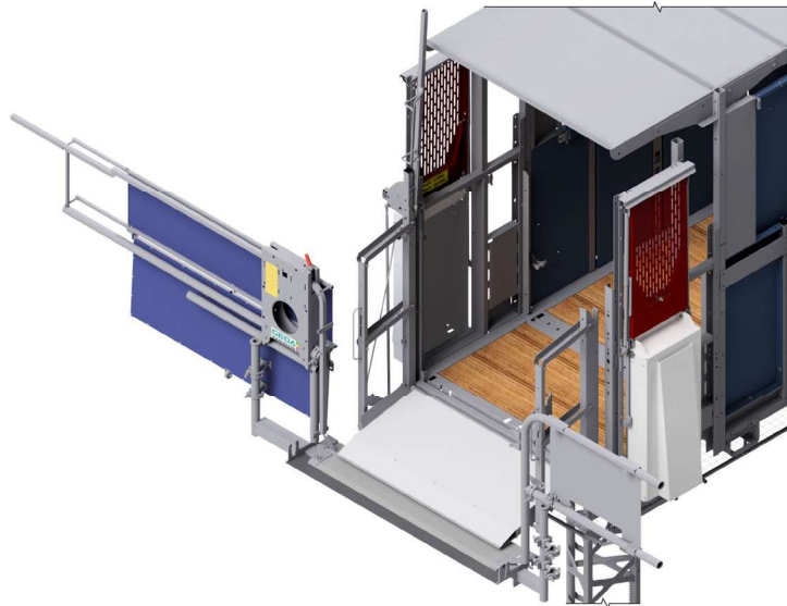
Abb. 51: Bühnenzugang Etage
