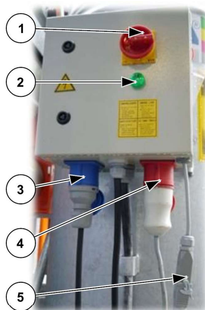
Abb. 34: Schaltkasten Bodenstation
