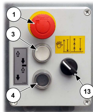
Abb. 77: Bodensteuerung für Umwendung (HAND)
