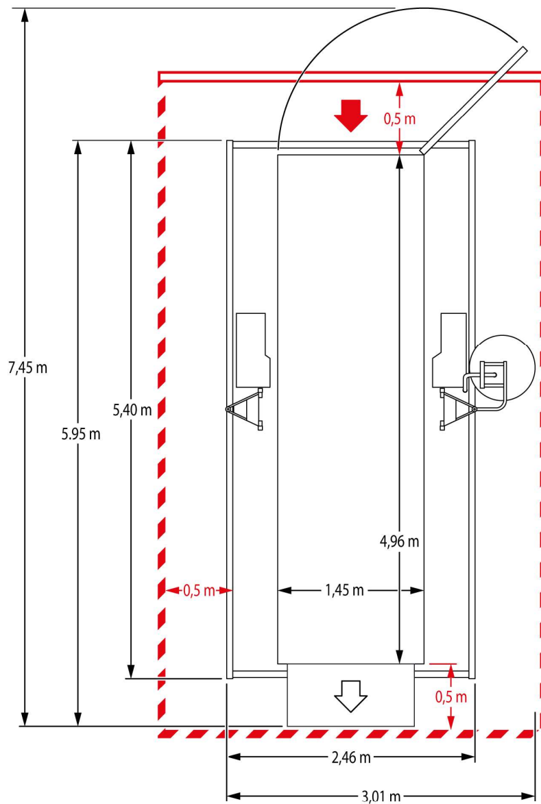
Abb. 11: Platzbedarf Bühne BLL
