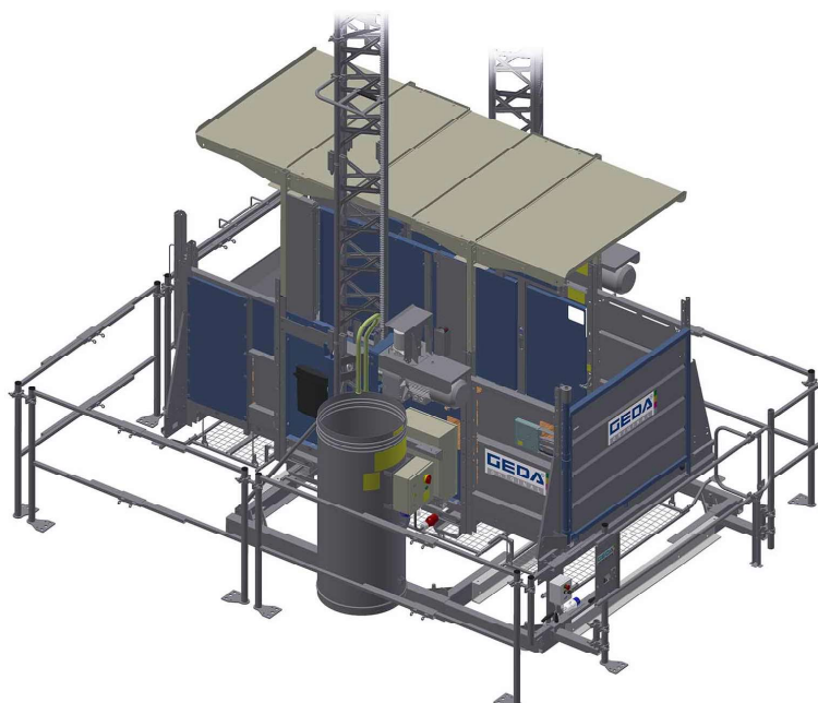
Abb. 38: Bodenumwehrung 1,10 m mit Schranke
