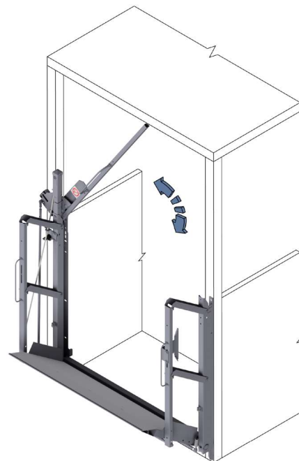
Abb. 56: Schranke mit elektromechanischer Verriegelung öffnen/schließen
