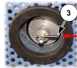
Abb. 46: Türschloss verriegelt
