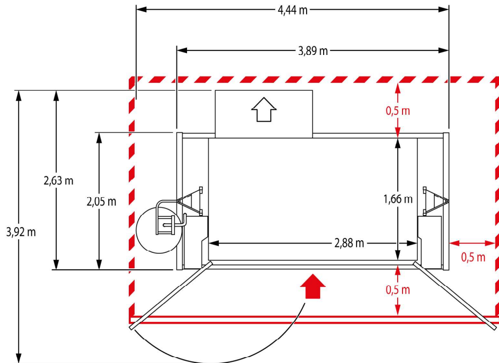
Abb. 15: Platzbedarf Bühne C
