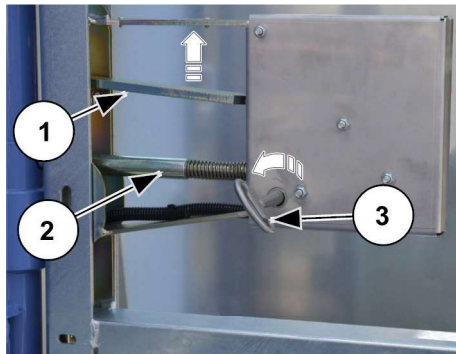
Abb. 48: Notentriegelung Rampe / Beladetür außen
