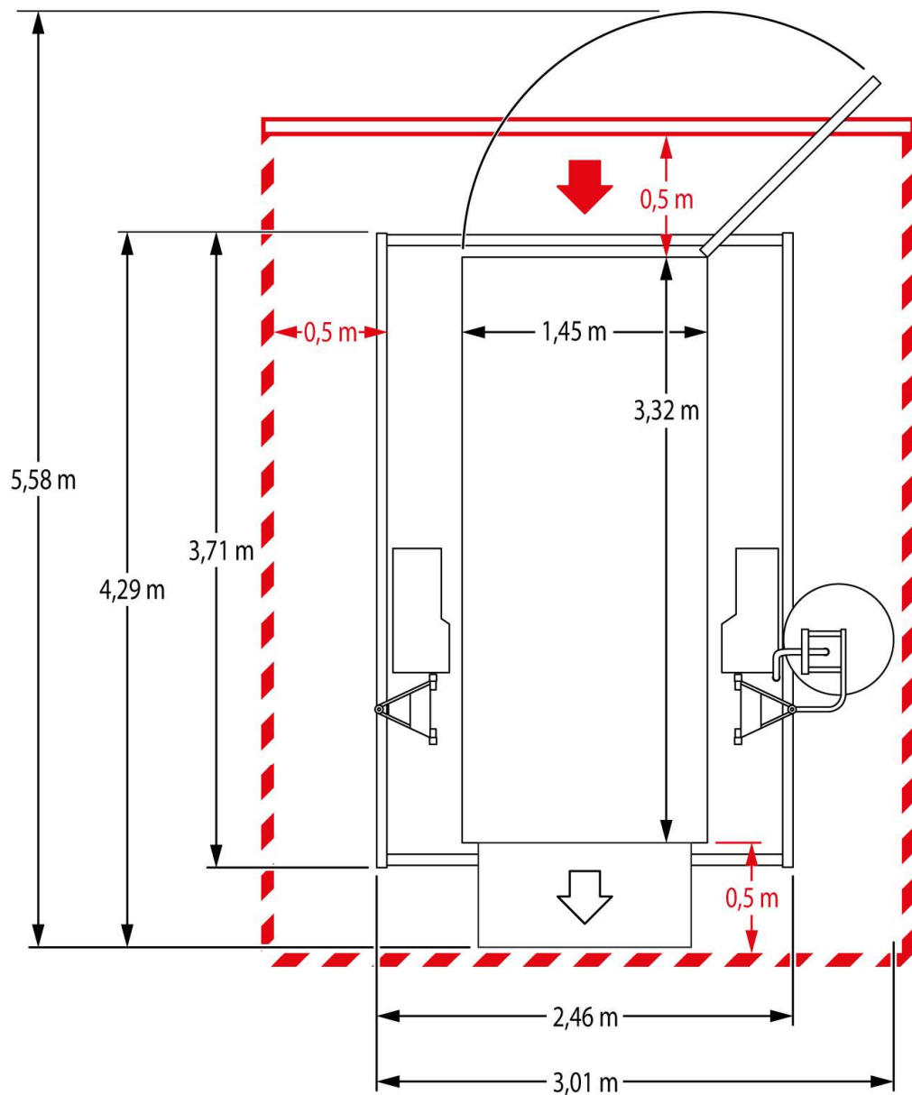
Abb. 7: Platzbedarf Bühne B
