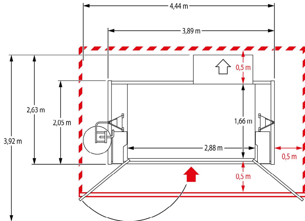
Abb. 17: Platzbedarf Bühne D
