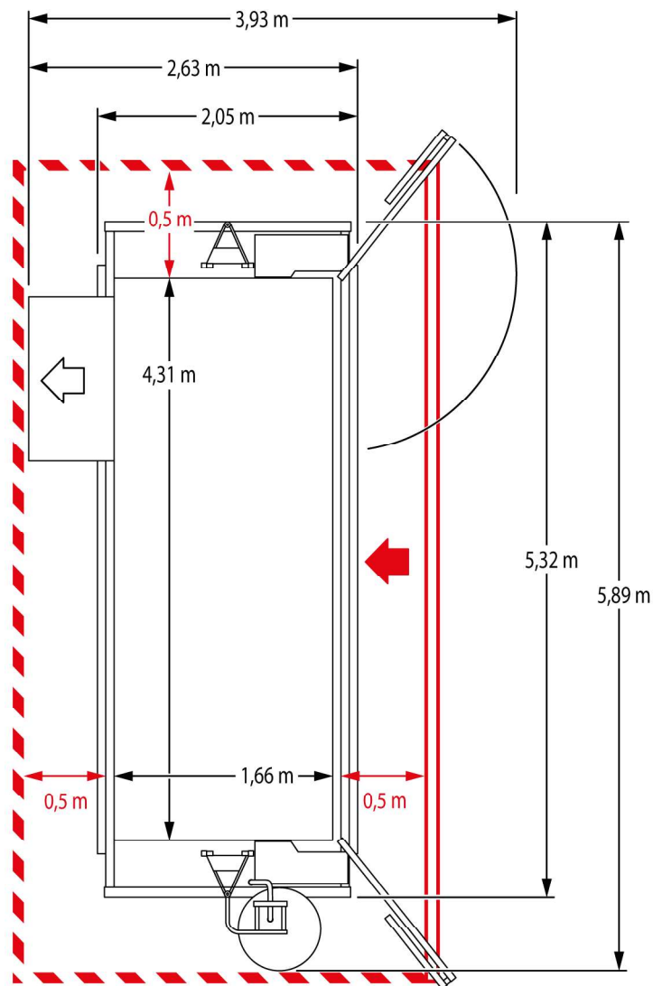
Abb. 27: Platzbedarf Bühne G
