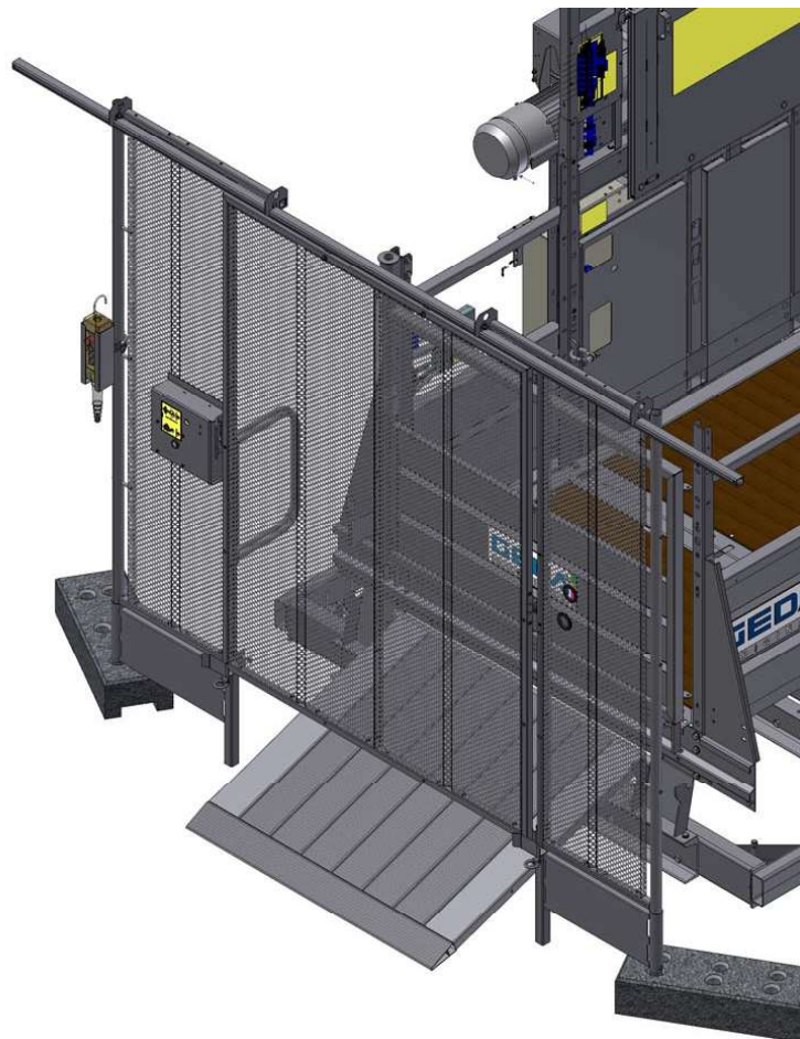
Abb. 39: Schiebetür für Bodenumweh rung geschlossen
