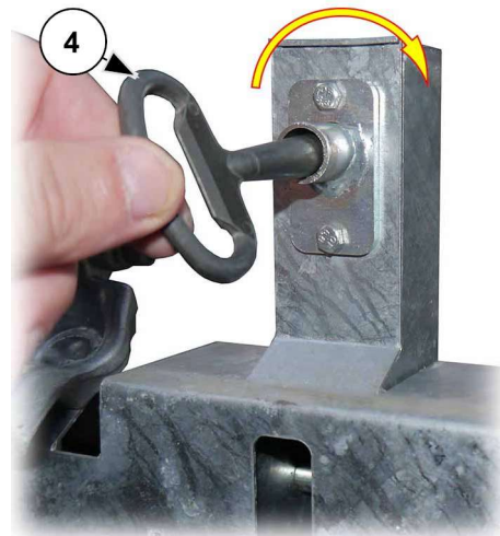
Abb. 74: Notentriegelung der Etagensicherungstür
