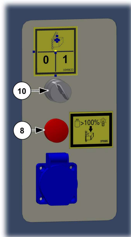
Abb. 101: Überlastanzeige
