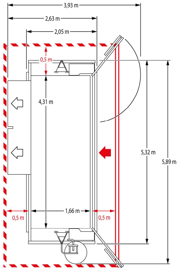
Abb. 29: Platzbedarf Bühne GD
