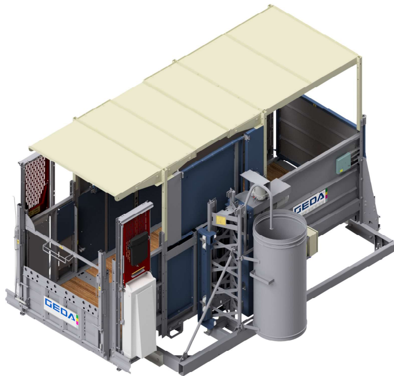
Abb. 8: Bühne BL
