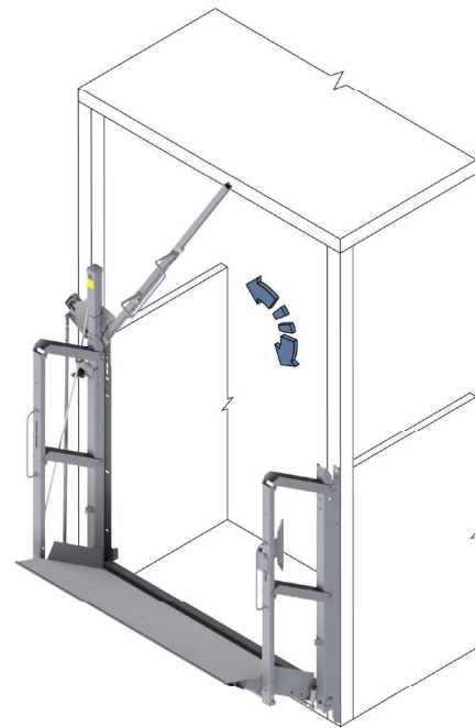
Abb. 54: Schranke mit mechanischer Verriegelung schließen
