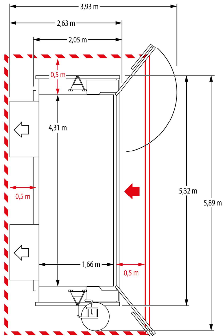
Abb. 31: Platzbedarf Bühne H
