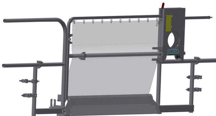
Abb. 67: Etagensicherungstür "Comfort" geschlossen (Plane)
