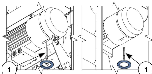
Abb. 109: Bremslufthebel in die Motorbremse einschrauben
