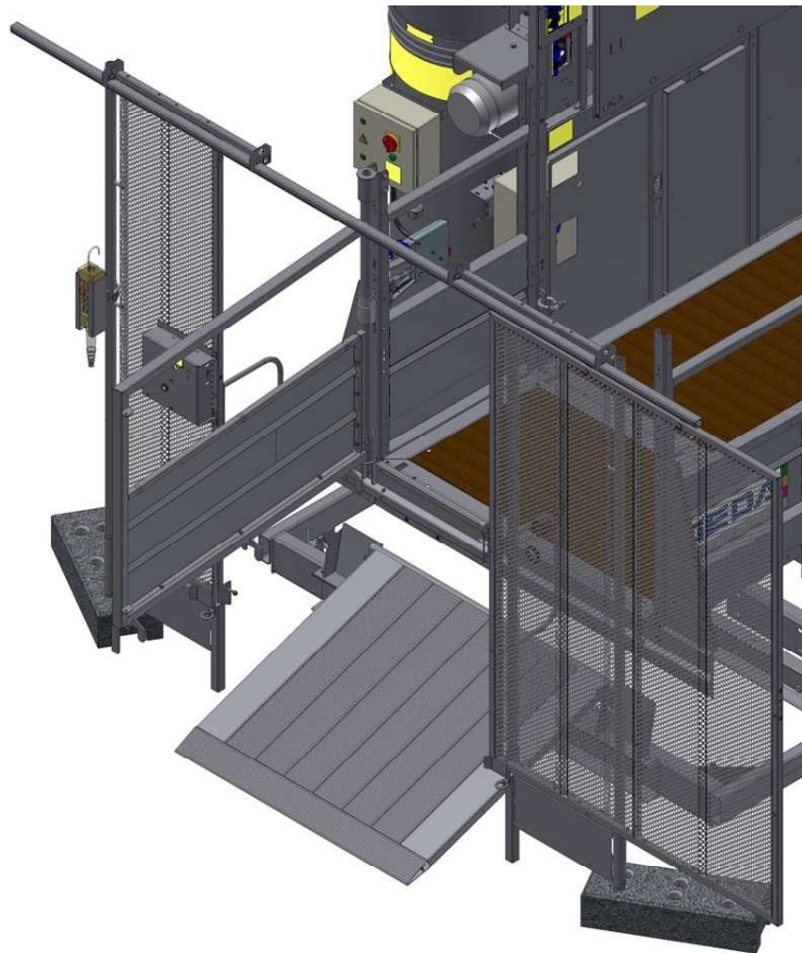
Abb. 43: Schiebetür für Bodenumwehrung geöffnet
