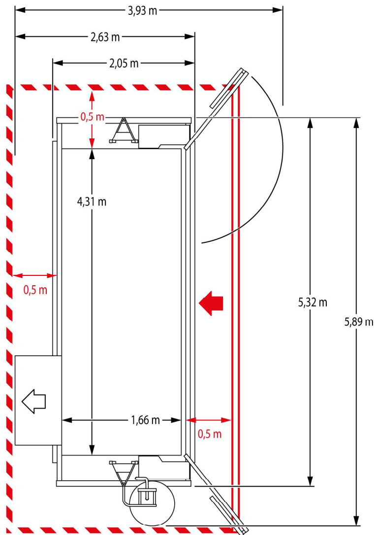
Abb. 25: Platzbedarf Bühne F
