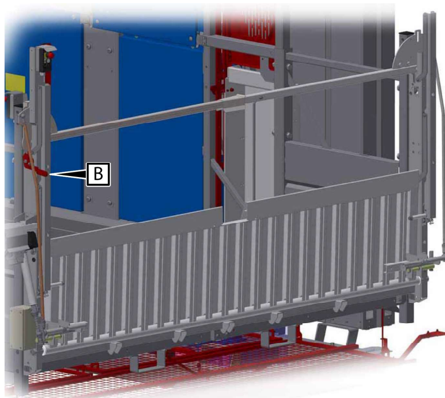
Abb. 60: E-Schranke mit Laderampe 2,82 m
