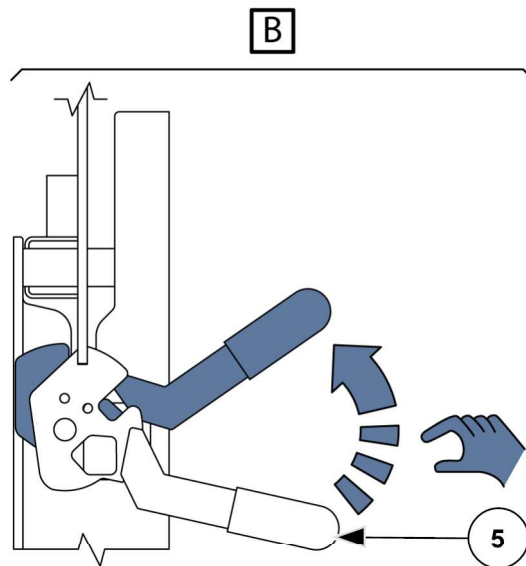
Abb. 61: Elektrisch angetriebene Laderampe entriegeln
