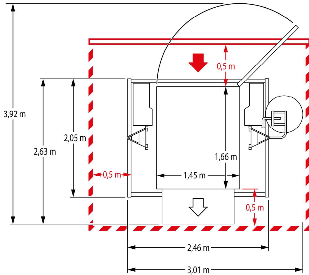
Abb. 5: Platzbedarf Bühne A
