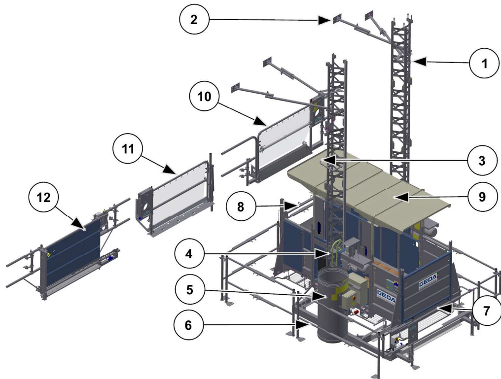
Abb. 36: Maschine Übersicht
