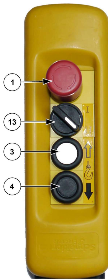
Abb. 78: Bodensteuerung/Handsteuerung (Stellung II)
