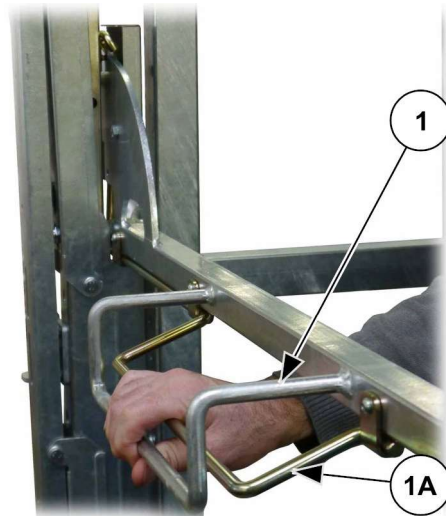
Abb. 53: Schranke mit mechanischer Verriegelung öffnen
