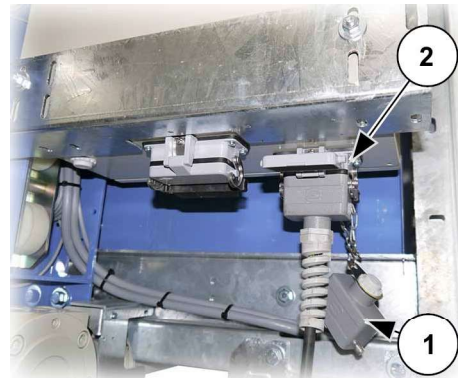
Abb. 102: Blindstecker Fangprobensteuerung
