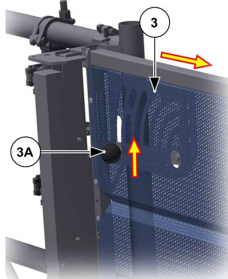
Abb. 73: Etagensicherungstür "VARIO" öffnen/schließen
