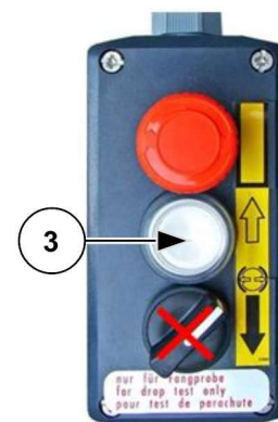
Abb. 103: Fangprobensteuerung
