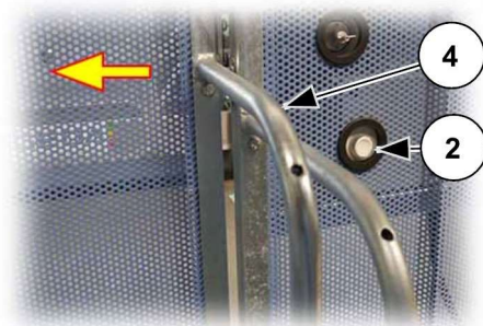
Abb. 41: Schiebetür öffnen
