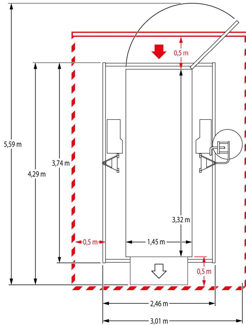
Abb. 13: Platzbedarf Bühne BS
