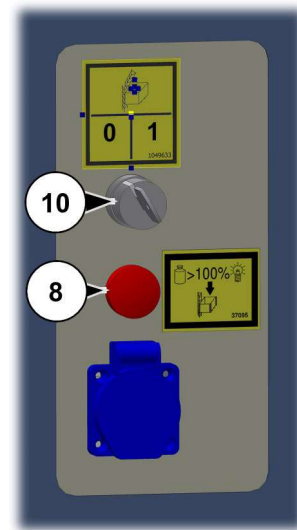
Abb. 35: Wahlschalter Betriebsart Betrieb
