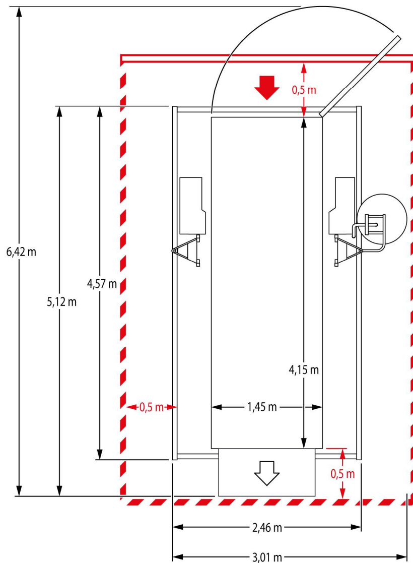
Abb. 9: Platzbedarf Bühne BL
