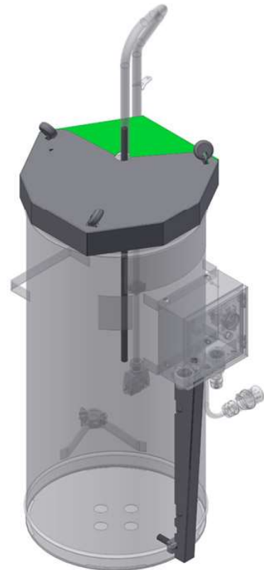
Abb. 95: Kabeltopfabdeckung
