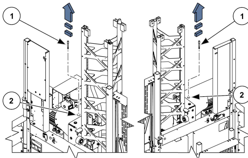
Abb. 108: Bremslufthebel aus der Halterung nehmen
