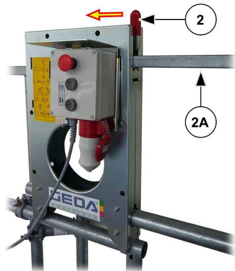
Abb. 70: Etagensicherungstür "Comfort" öffnen/schließen
