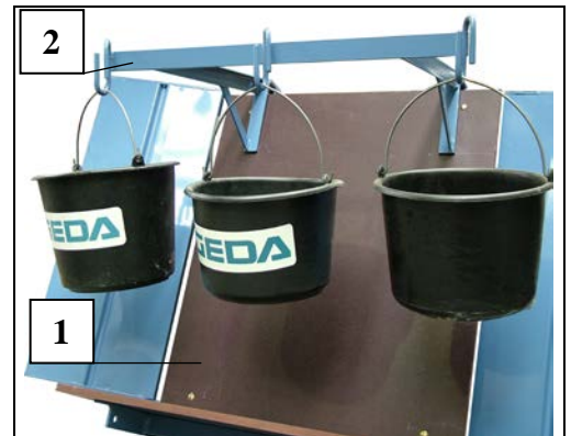
Fig. 44 Eimergehänge
