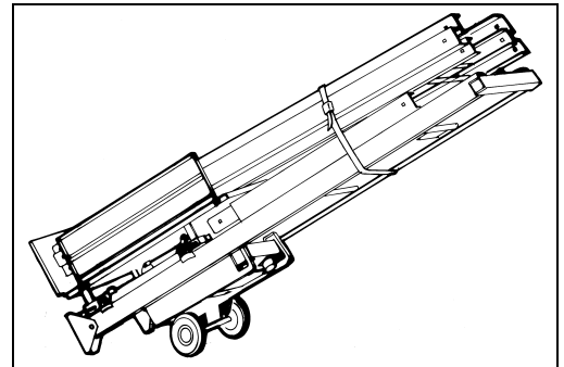
Fig. 12 Fahrgestell
