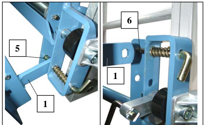
Fig. 42 Universalpritsche montieren
