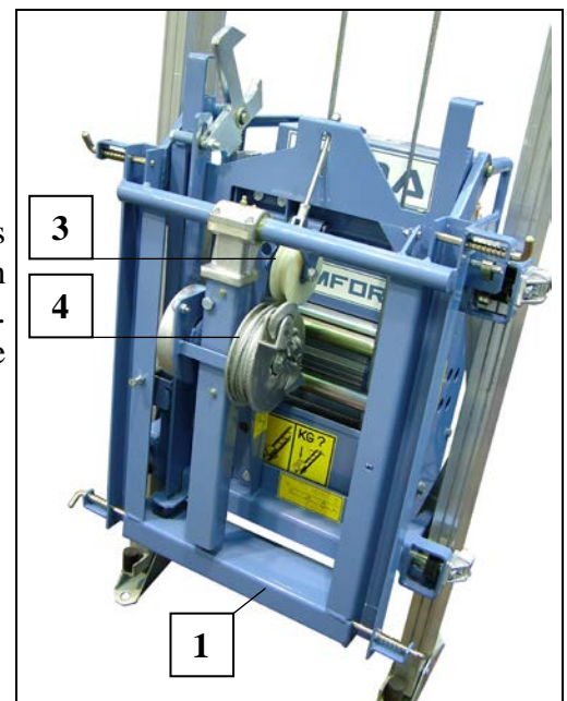
Fig. 63 Kippschlitten
