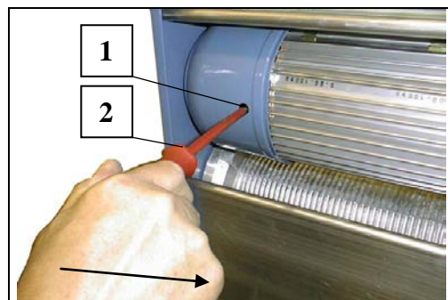
Fig. 73 Bremse lüften
