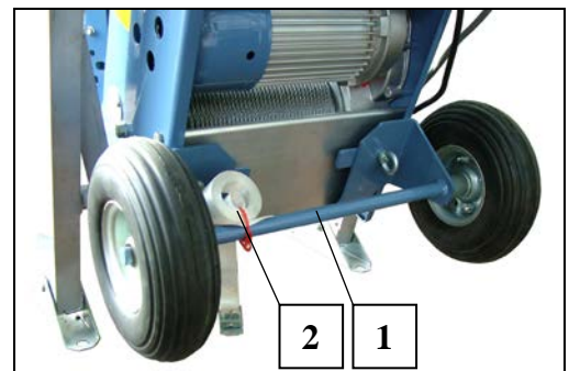
Fig. 13 Fahrgestell montieren
