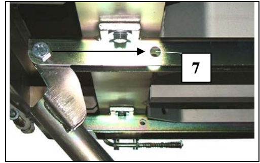
Fig. 52 Teleskopstützen abstecken
