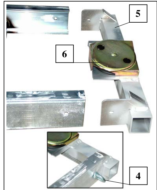
Fig. 20 Kopfstück montieren
