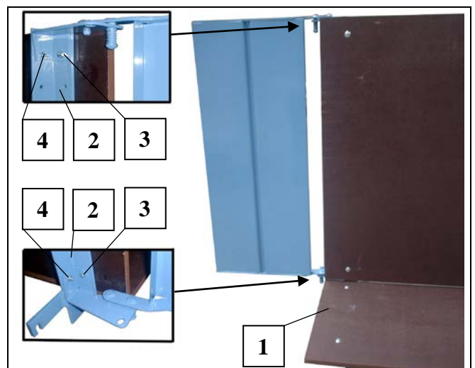
Fig. 40 Universalpritsche zusammenbauen
