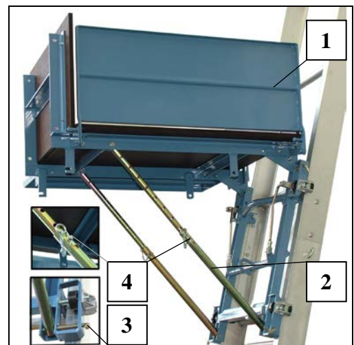
Fig. 47 Vario- Bühne
