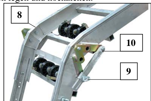
Fig. 22 Knickstück einstellen
