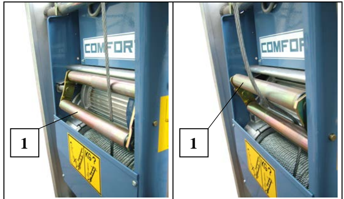
Fig. 11 Endschalter unten
