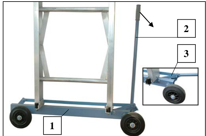
Fig. 14 Fahrwerk
