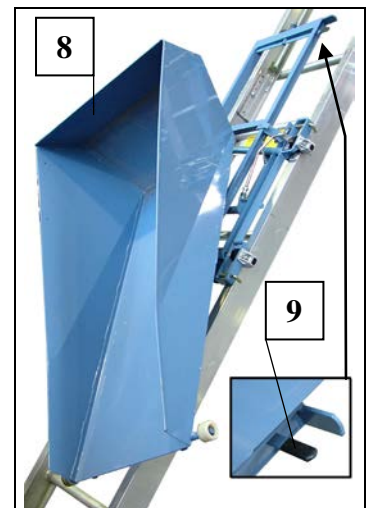
Fig. 62 Kippmulde entleeren
