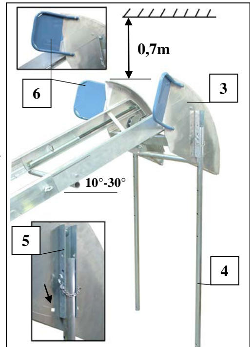
Fig. 60 Kippvorrichtung
