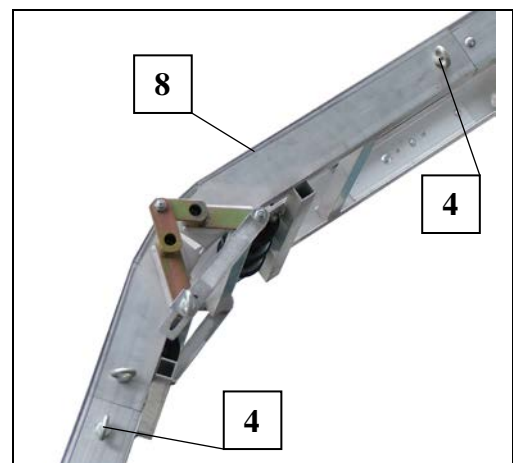
Fig. 21 Knickstück montieren
